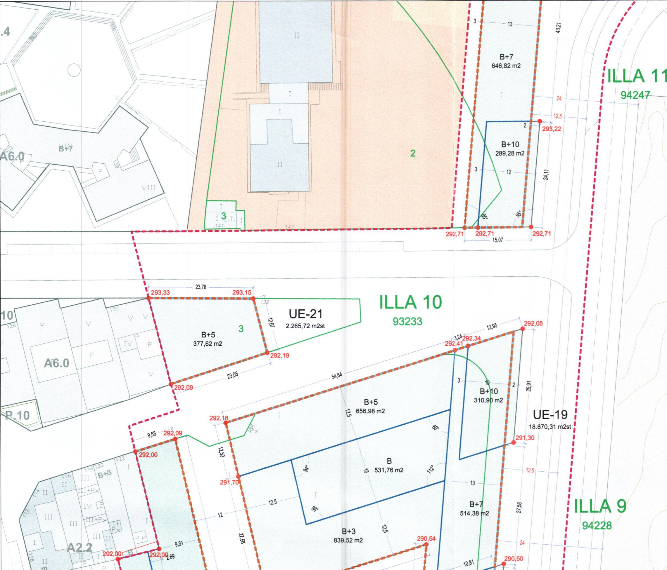
PLANTA SOTERRANI
